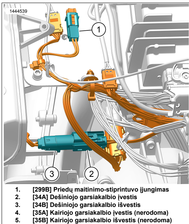
Pav 2. Ant rėmo montuojamo garsiakalbio kabelis (rodoma dešinė pusė, kairė - panaši)
