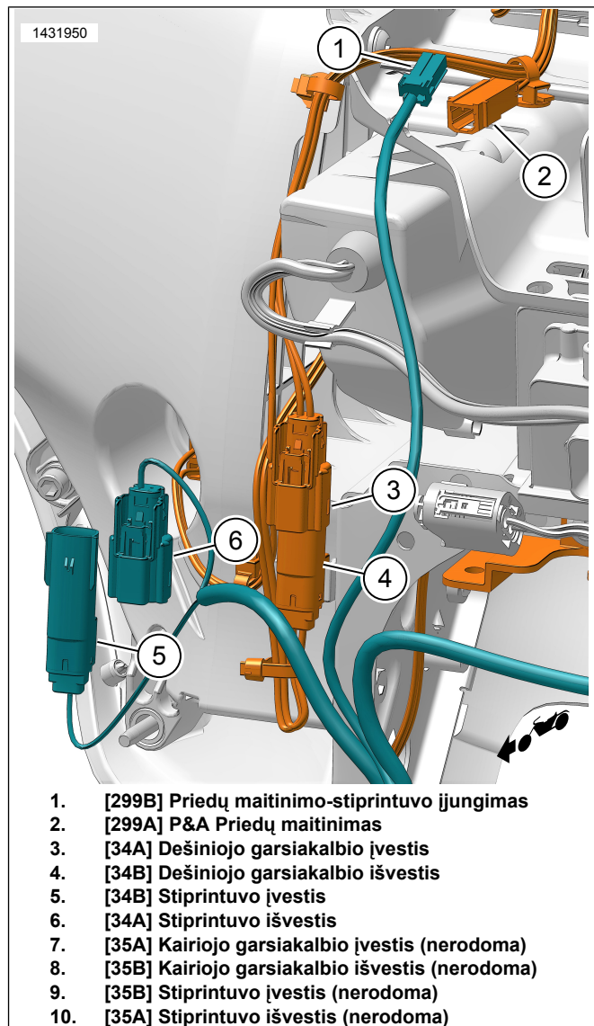
Pav 1. Ant šakės montuojamas garsiakalbio kabelis (rodoma dešinė pusė, kairė - panaši)
