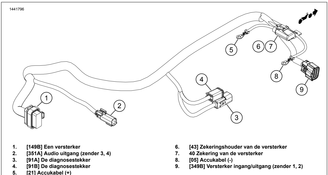
Afbeelding 4. Kabelboom van versterker (2014-2016 modellen)
