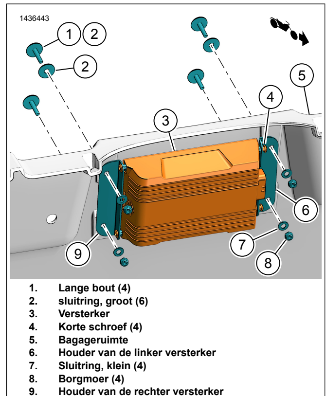
Afbeelding 2. Steunhouder voor de versterker
