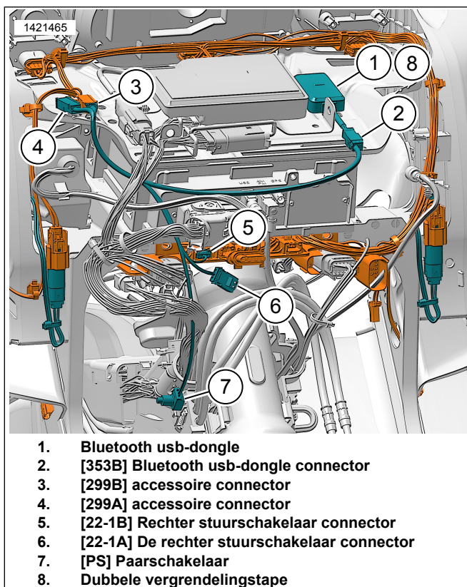
Afbeelding 6. Op de vork gemonteerde kuip met bluetooth usb-dongle kabelboom (2014 en latere modellen)
