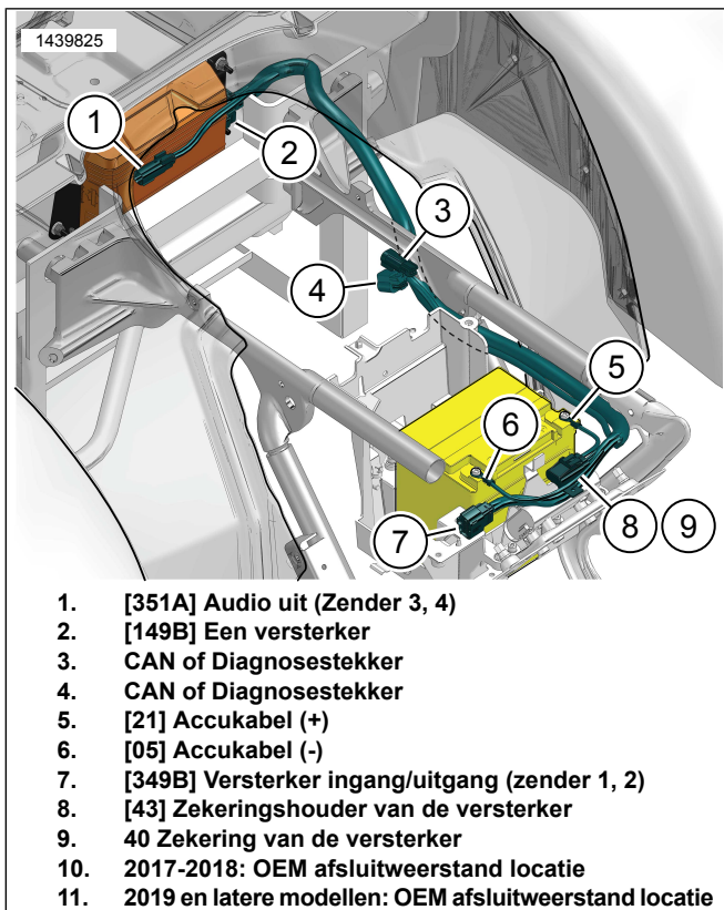
Afbeelding 3. Verloop van de kabelboom van de versterker
