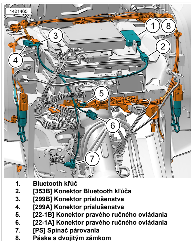
Obrázok 6. Zväzok Bluetooth kľúča kapotáže pripevnenej k vidlici (2014 a novšie)
