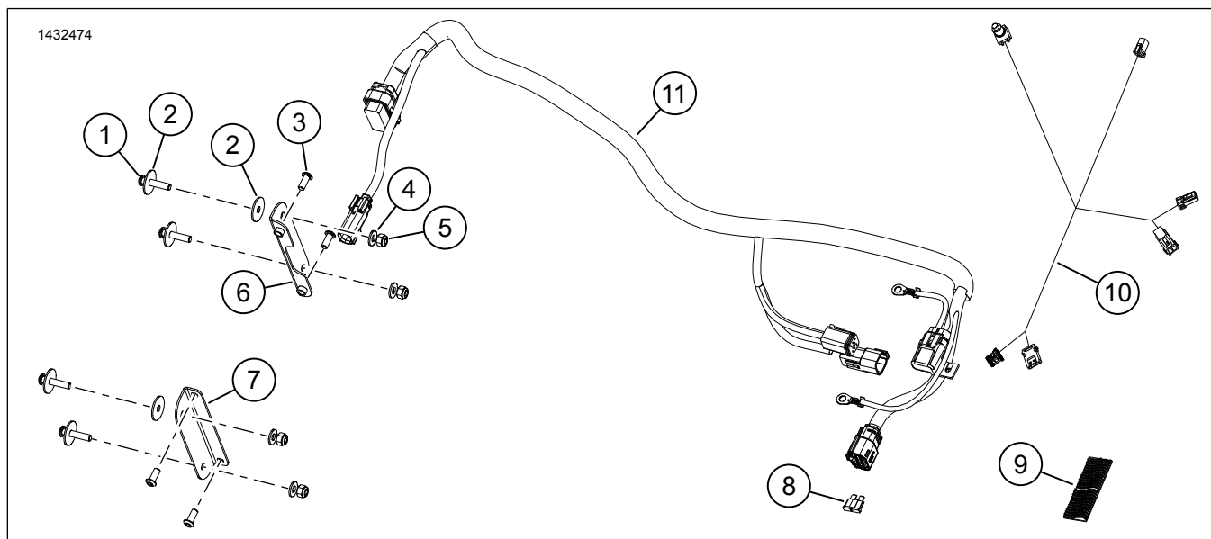
Obrázok 1. Servisné diely: Súprava primárneho zosilňovača
