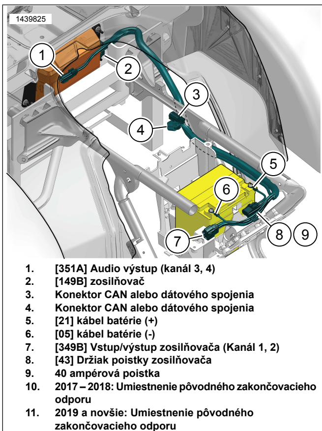
Obrázok 3. Trasa zväzku káblov zosilňovača
