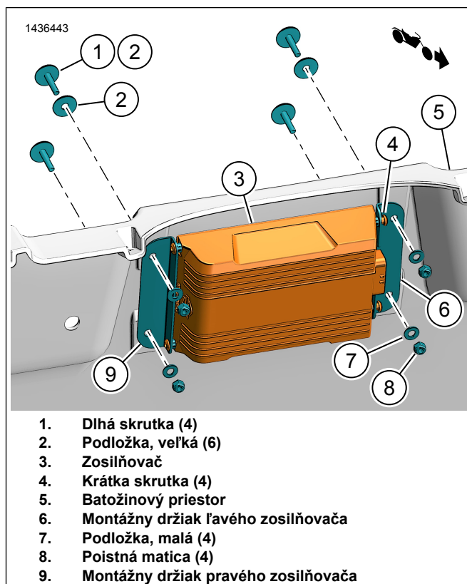
Obrázok 2. Montážne držiaky zosilňovača
