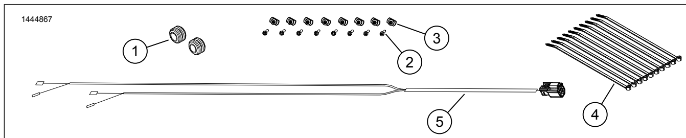
Figura 3. Parti di ricambio, altoparlanti per carenatura inferiore
