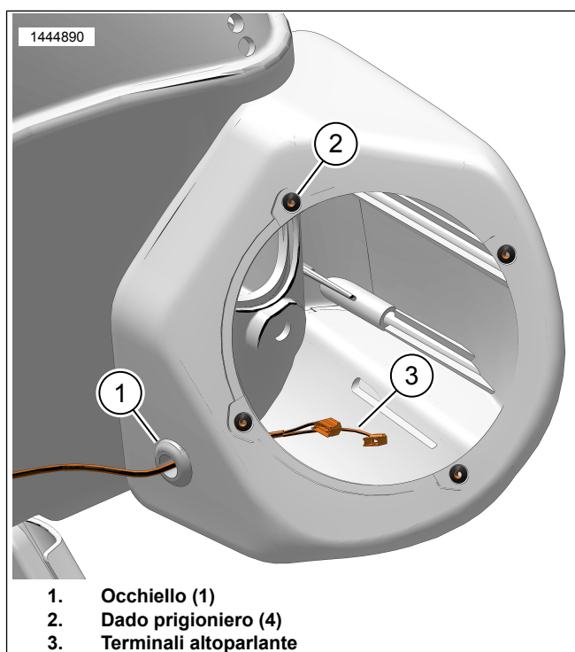
Figura 1. Cablaggio guscio altoparlante (mostrato il lato sinistro)
