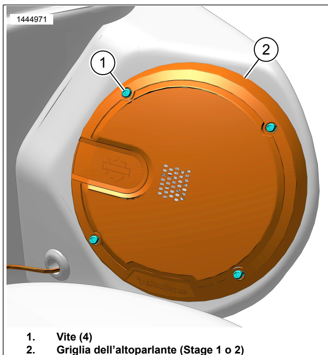
Figura 2. Griglia per guscio dell'altoparlante (mostrato il lato sinistro)
