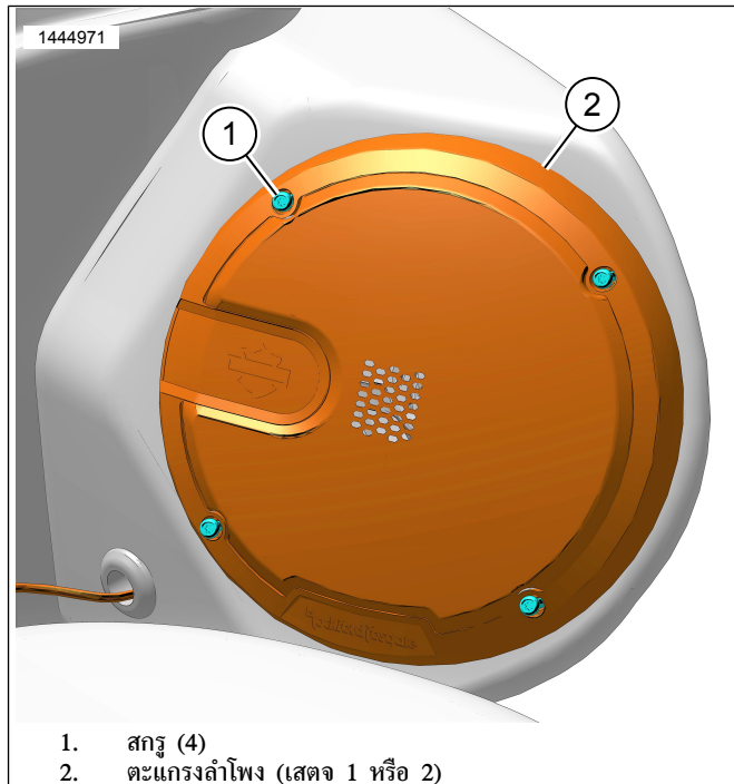
รูปภาพ 2 ตะแกรงตู้ลำโพง (แสดงด้านซ้าย)
