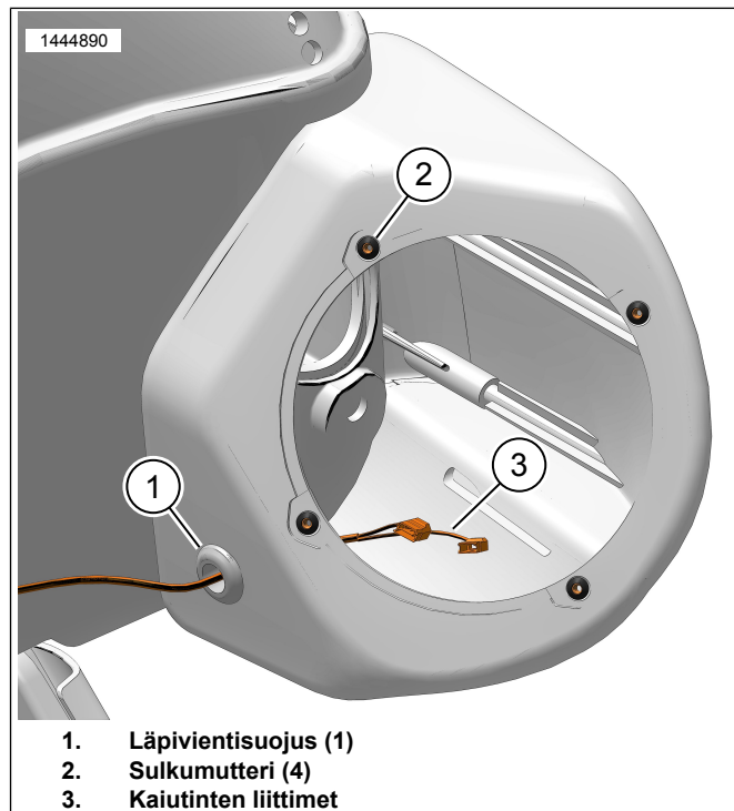
Kuva 1. Kaiutinkotelon johtosarja (vasenpuoli kuvassa)
