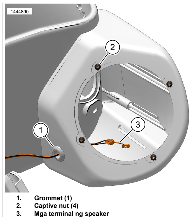
Figure 1. Speaker Pod Wire Harness (Kaliwang Panig ang Ipinakikita)
