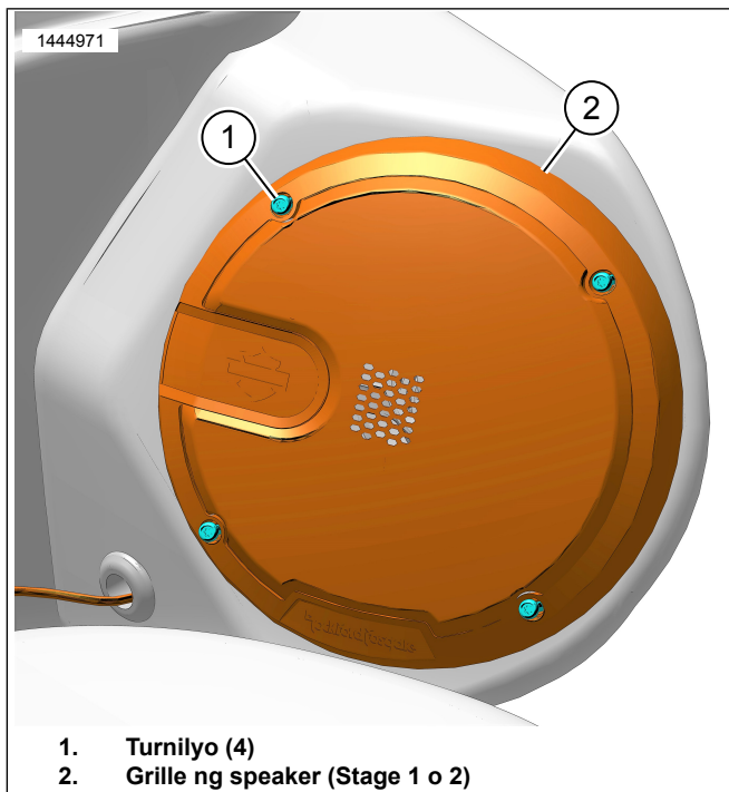
Figure 2. Speaker Pod Grille (Kaliwang Bahagi Ang Ipinakikita)
