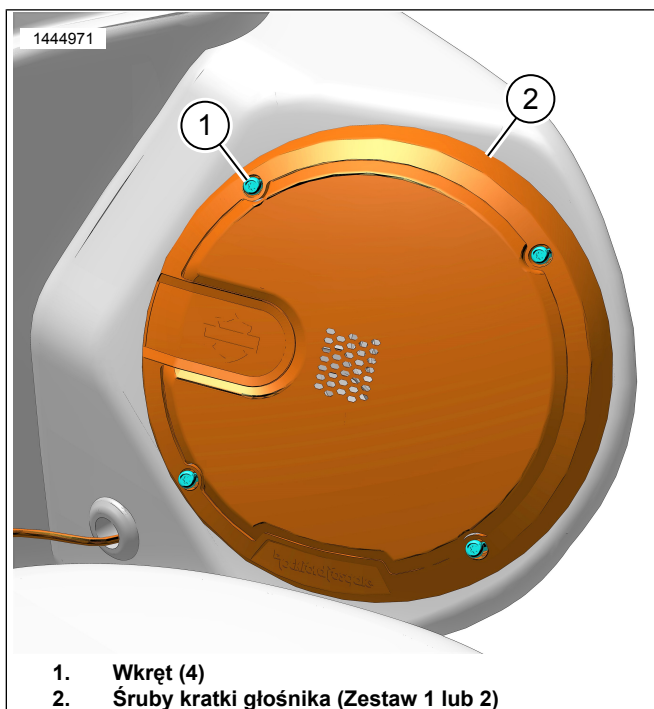
Rysunek 2. Kratka głośnika (na ilustracji pokazano lewą)
