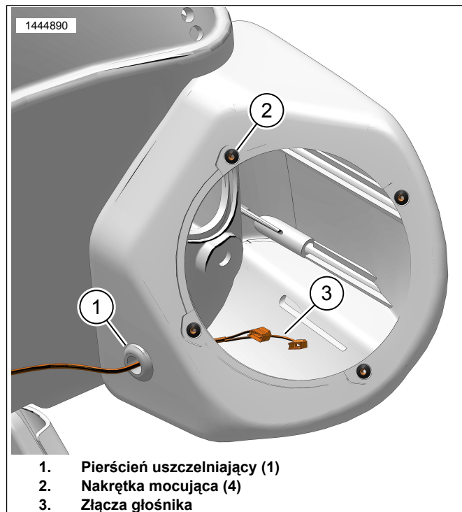
Rysunek 1. Wiązka przewodów obudowy głośnika (na ilustracji pokazano lewą)
