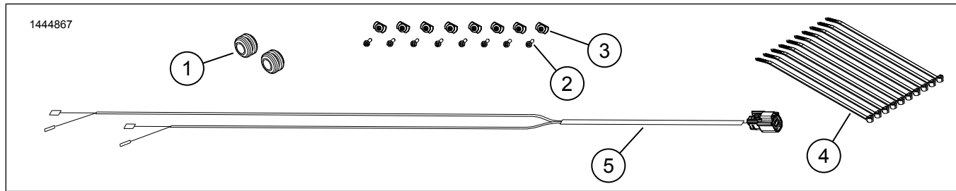
Afbeelding 3. Serviceonderdelen, Onderkuipluidsprekers
