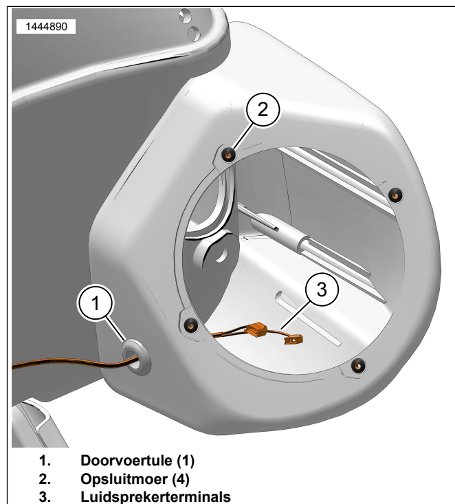
Afbeelding 1. Kabelboom luidsprekerhuls (linkerzijde weergegeven)
