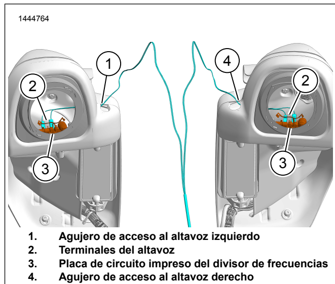
Figura 1. Arnés de cables del altavoz
