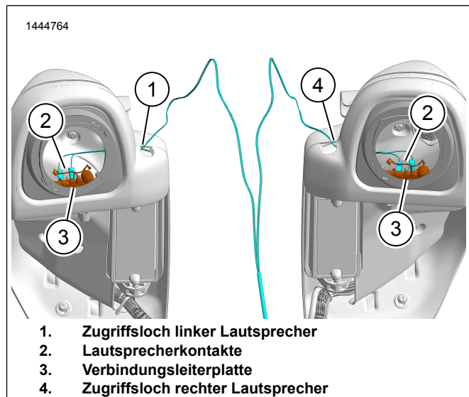
Abbildung 1. Lautsprecherkabelbaum
