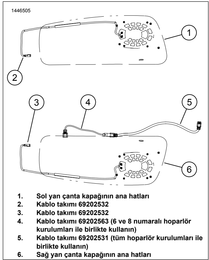
Şekil 6. Kablo Takımının Kurulumu ve Çekilmesi
