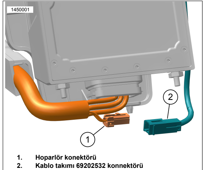
Şekil 7. Sol Yan Çanta Hoparlör Bağlantısı, Sağ ile Aynıdır
