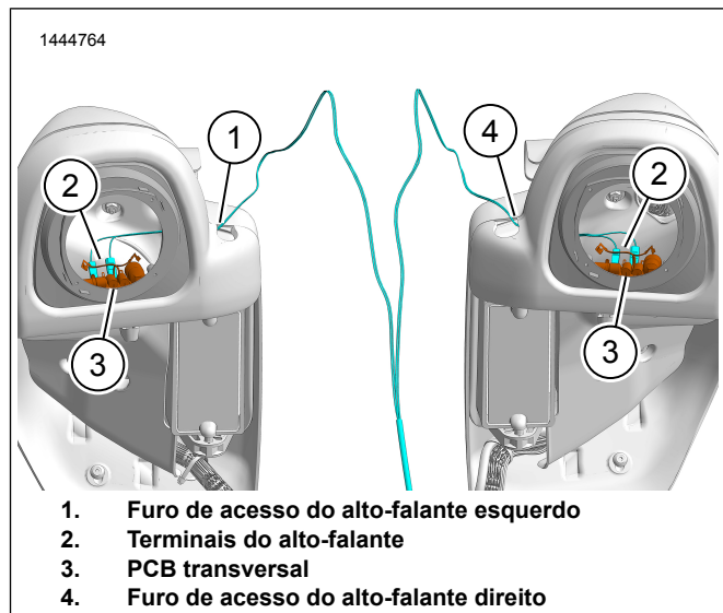
Figura 1. Chicote de fios do alto-falante
