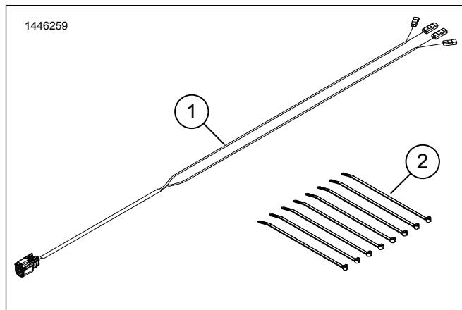
Figura 2. Peças de serviço, alto-falantes da carenagem inferior
