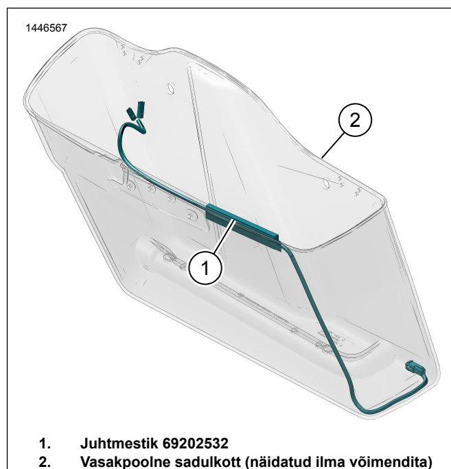
Joonis 4. Vasakpoolse sadulakoti juhtmekimbu paigutus
