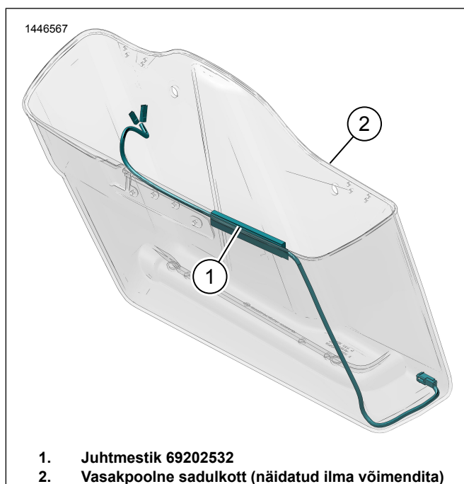
Joonis 8. Vasakpoolse sadulakoti juhtmestiku paigutus
