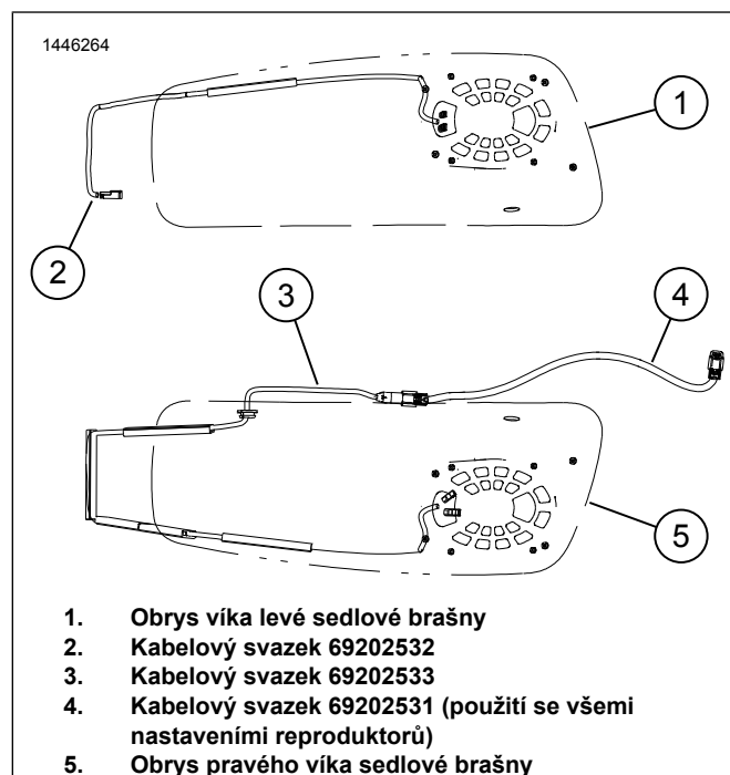
Ilustrace 2. Nastavení a vedení kabelového svazku
