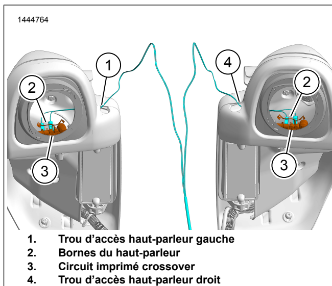
Figure 1. Faisceau de fils de haut-parleur
