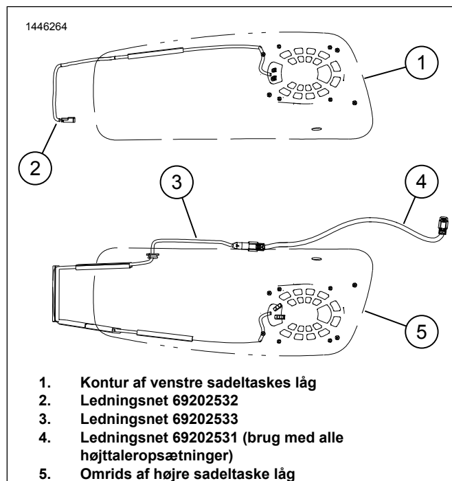
Figur 2. Ledningsopsætning og føring
