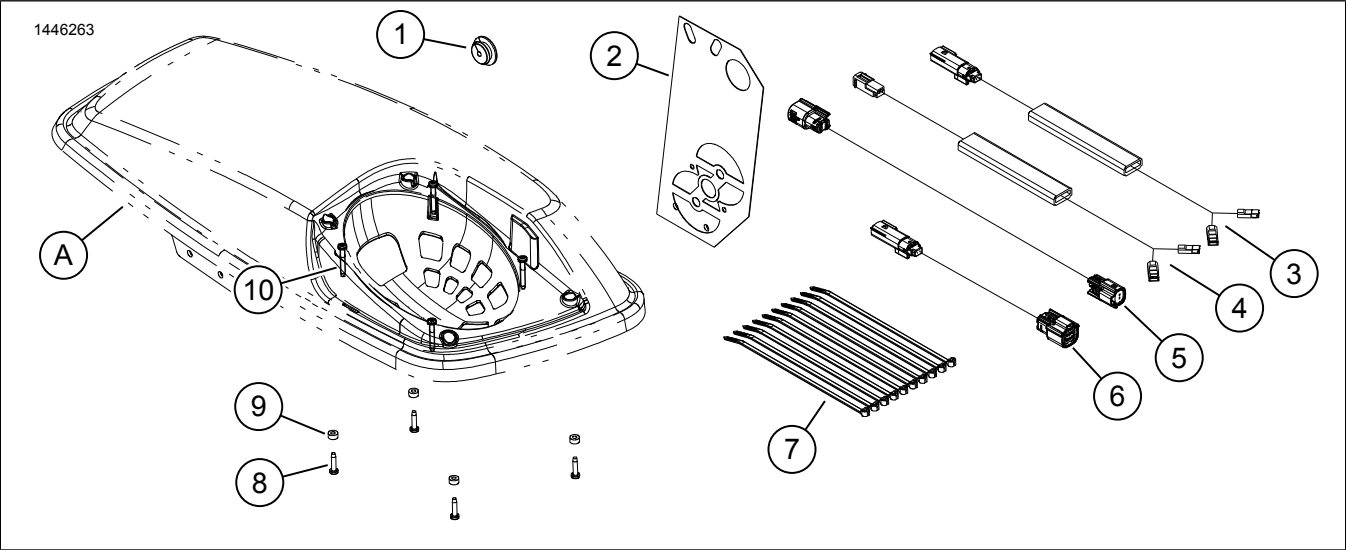
Figur 10. Servicedele, højttalere med nedre strømlinjebeklædning
