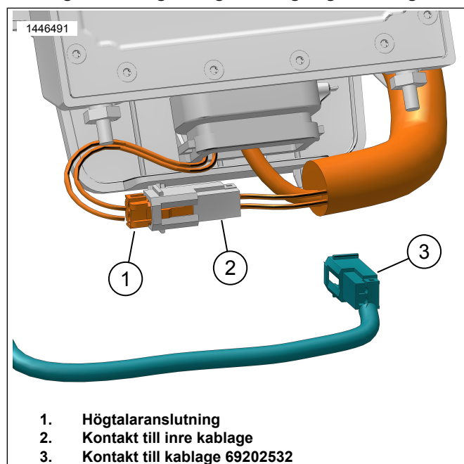
Figur 3. Vänstra packväskeshögtalarens anslutning
