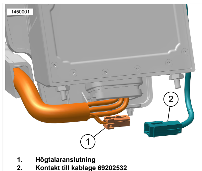
Figur 7. Vänstra packväskenhögtalarens anslutning, högra är liknande
