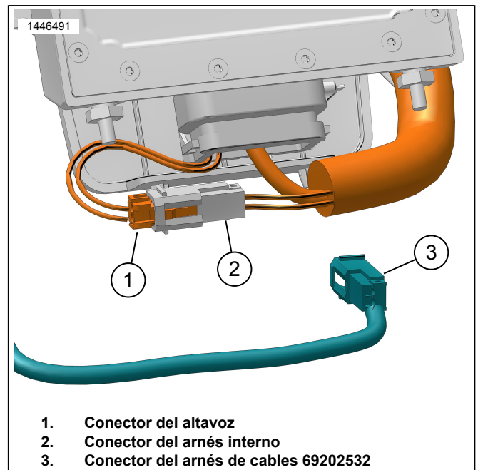
Figura 3. Conexión del altavoz de la alforja izquierda
