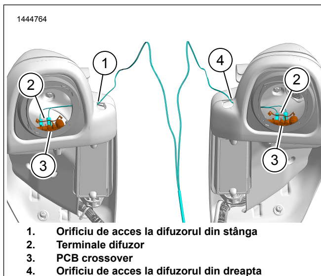
Figura 1. Cablaj difuzor
