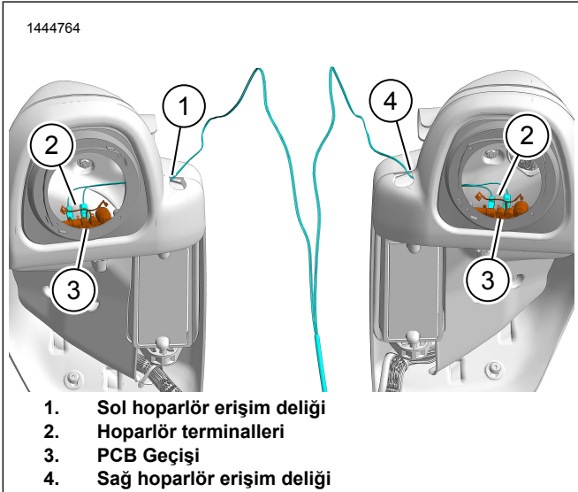
Şekil 1. Hoparlör Kablo Takımı
