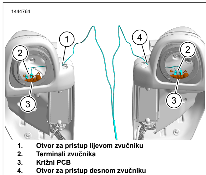
Slika 1. Kabelski snop zvučnika
