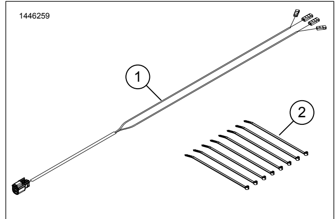
Slika 2. Servisni dijelovi, zvučnici u donjoj maski
