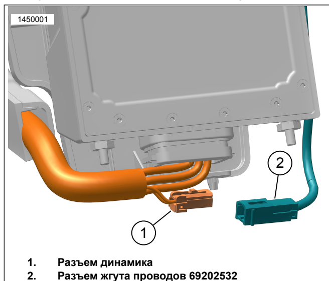
Рисунок 7. Соединение динамика левого кофра, правое аналогично
