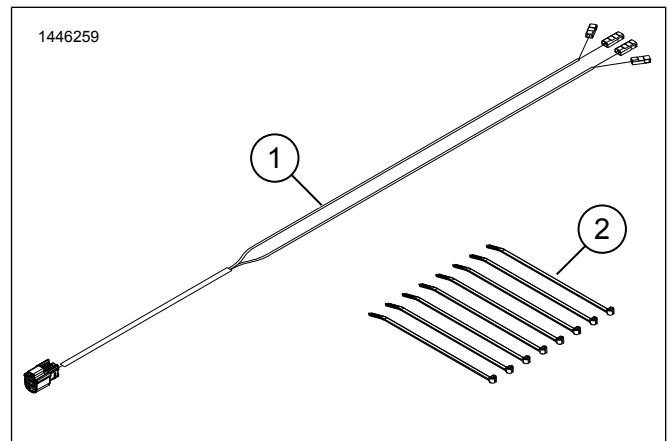
Figur 2. Servicedele, højttalere med nedre strømlinjebeklædning
