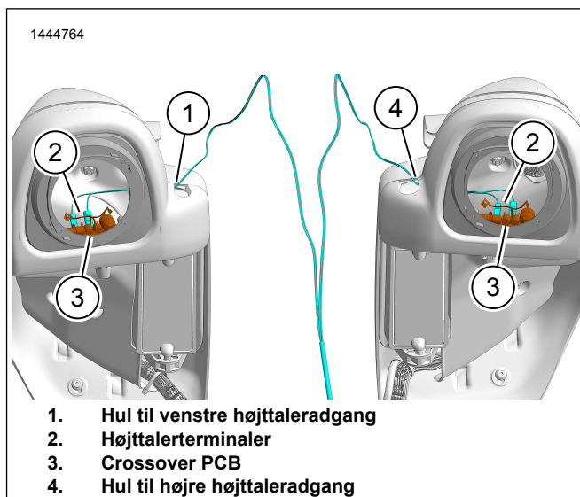
Figur 1. Ledningsnet til højttaler
