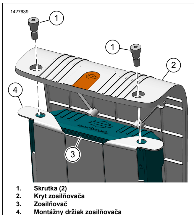
Obrázok 16. Kryt zosilňovača
