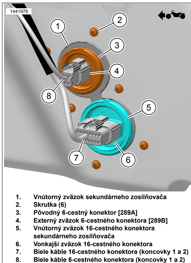
Obrázok 8. Biele káble vonkajšieho zväzku (vonkajšia strana sedlovej tašky)
