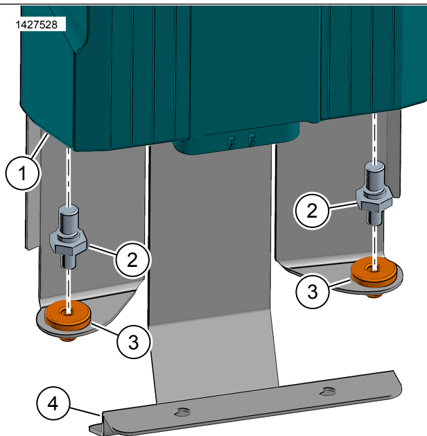
Obrázok 11. Inštalácia montážneho držiaka
