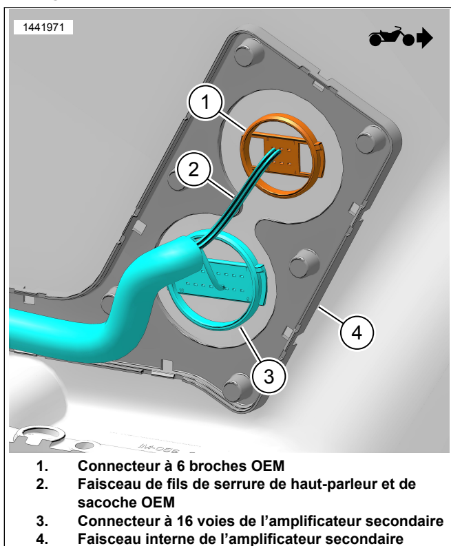
Figure 7. Faisceau interne de l'amplificateur secondaire (sacoche interne)
