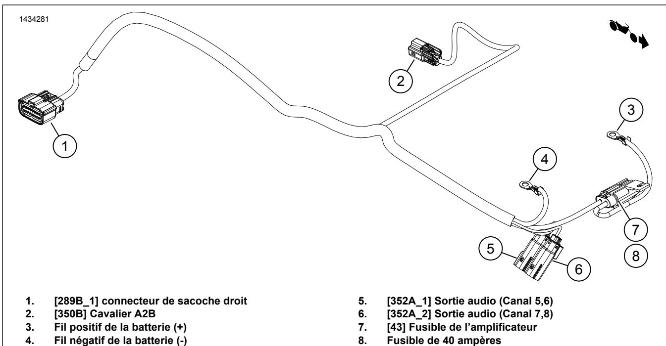
Figure 19. Connecteurs de faisceau externes (2014 et ultérieur)
