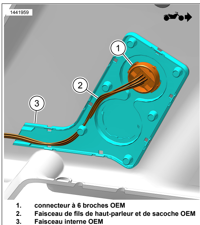
Figure 6. Faisceau interne OEM (sacoche interne)
