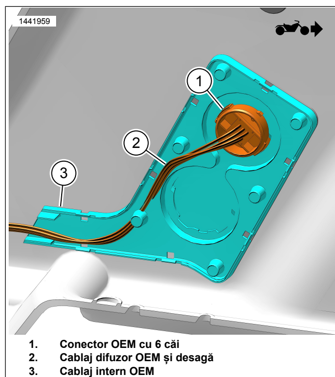
Figura 6. Cablaj intern OEM (interior desagă)
