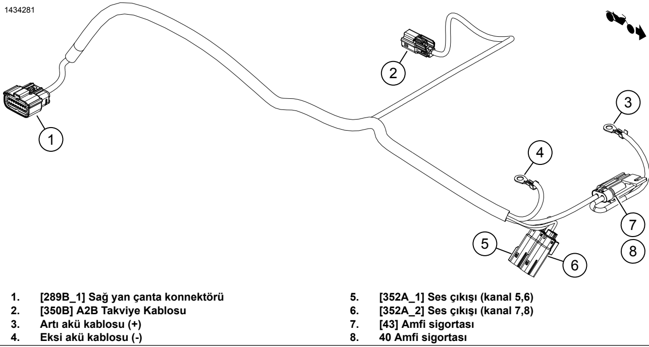
Şekil 19. Harici Kablo Takımı Konektörleri (2014 ve Sonrası)
