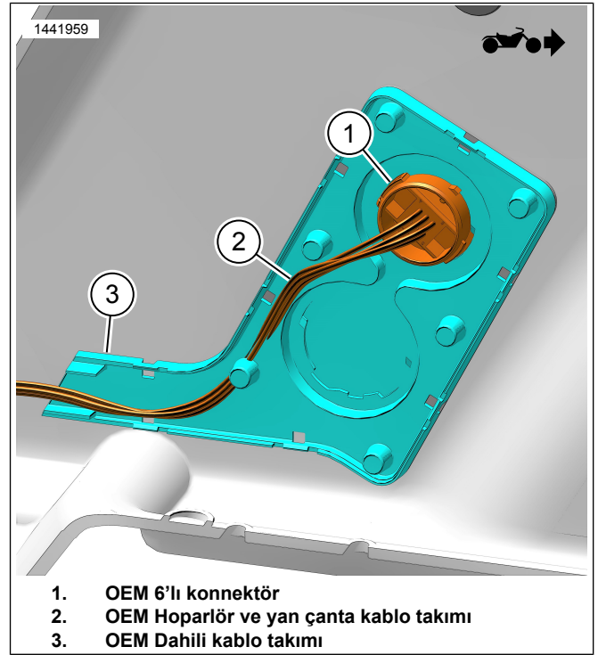
Şekil 6. OEM Dahili Kablo Takımı (Yan Çantanın İçinde)
