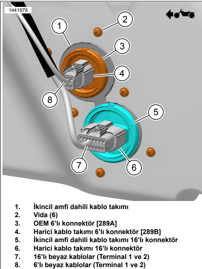
Şekil 8. Harici Kablo Takımı - Beyaz Kablolar (Yan Çantanın Dışında)
