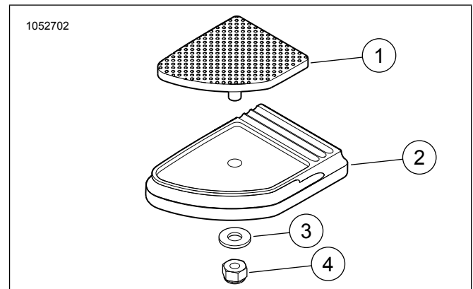
Figura 1. Piezas de servicio: Kit de almohadilla del pedal del freno pequeño
