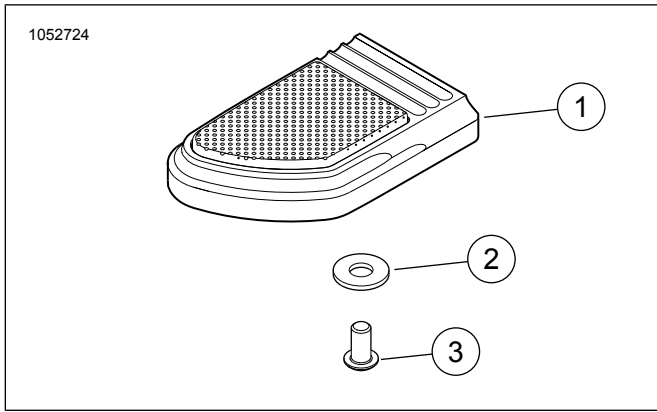
Figura 2. Piezas de servicio: Kit de almohadilla del pedal del freno grande
