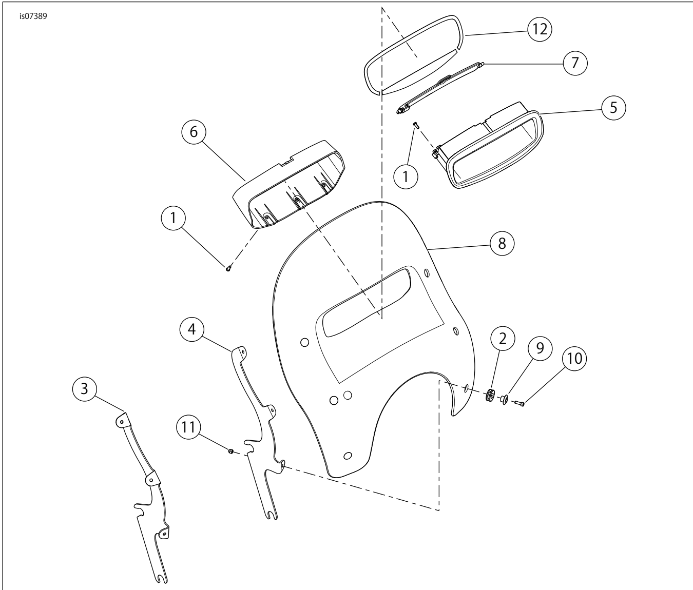
図1。交換用パーツ：ベンテッドデタッチャブルウィンドシールド
