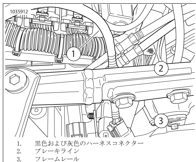
図12。灰色および黒色のコネクターハーネスの取り直し
