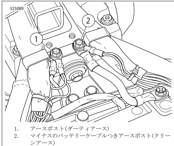
図34. バッテリーボックスのアースポストの位置
