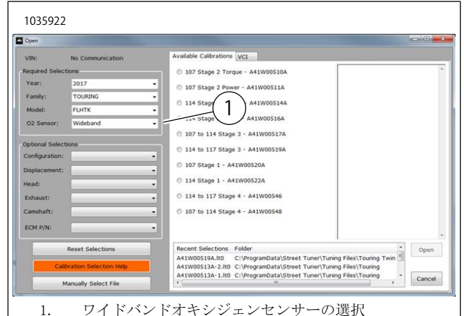
図37. ワイドバンドオキシジェンセンサーの選択
