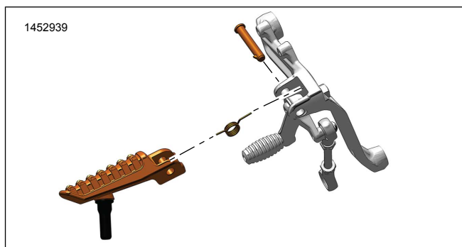
図4。フットペグ-ライダー-左
