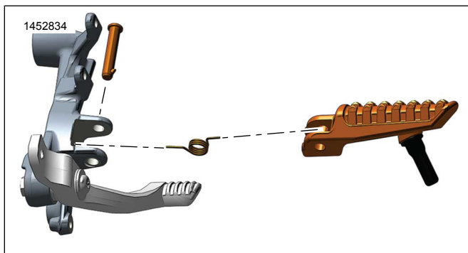
図3。フットペグ-ライダー-右
