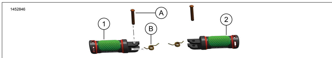
図1。キット内容: ADVERSARY フットペグ-ライダー
