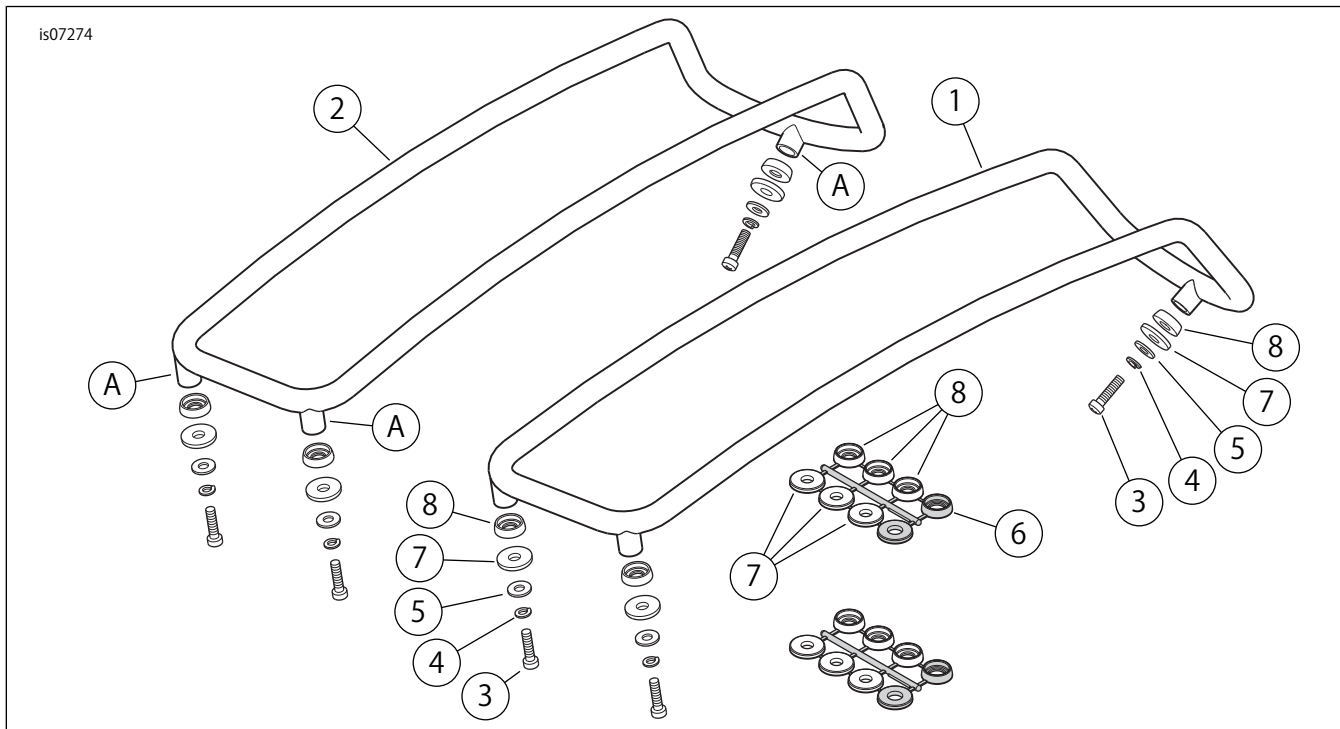
図1。交換用パーツ、ツーリングサドルバッグリッドレールキット
