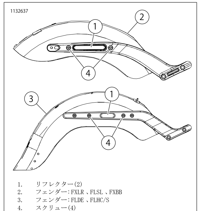
図1. フェンダーストラットスクリュー
