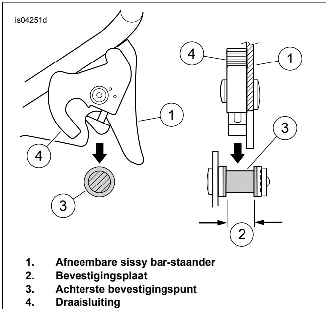
Afbeelding 1. Correcte uitlijning van de sluiting in het achterste bevestigingspunt, gezien vanuit de richting van de pijlen (D) en (E)
