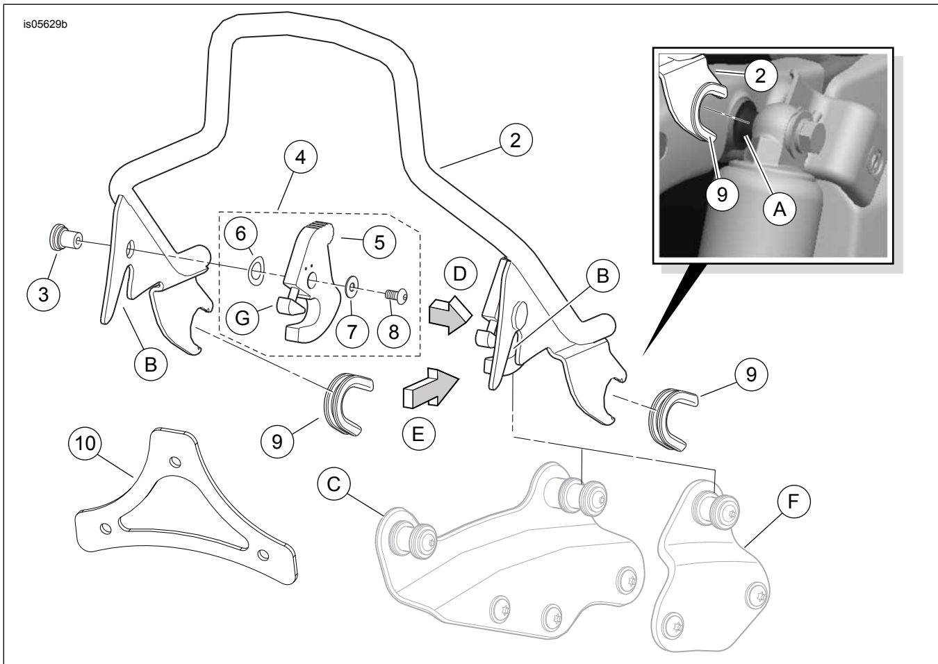
Afbeelding 3. Serviceonderdelen: H-D Detachables Touring sissy bar-standers
