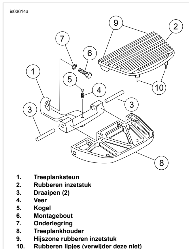
Afbeelding 1. Standaard treeplankmontage
