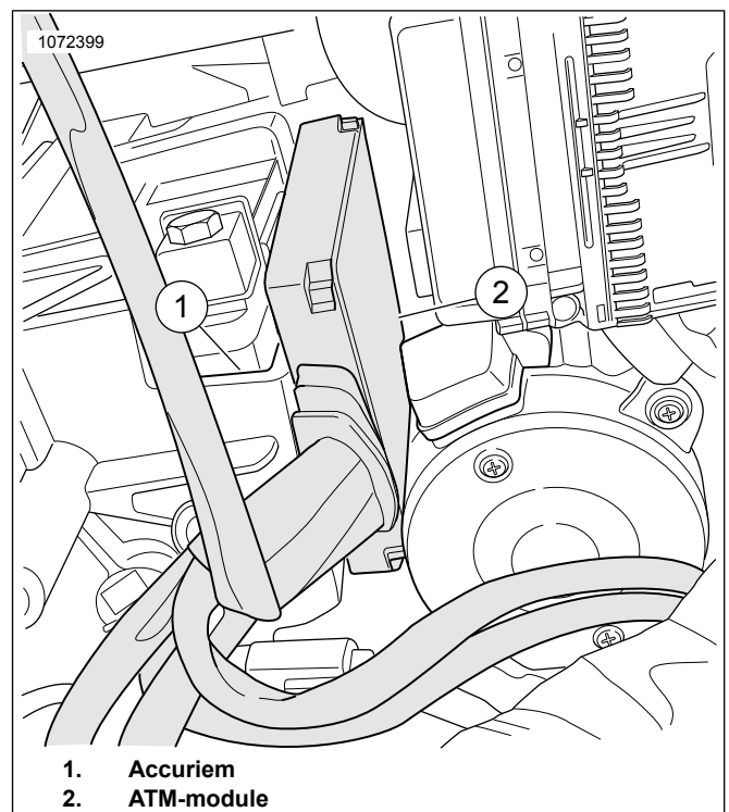
Afbeelding 18. Module plaatsen
