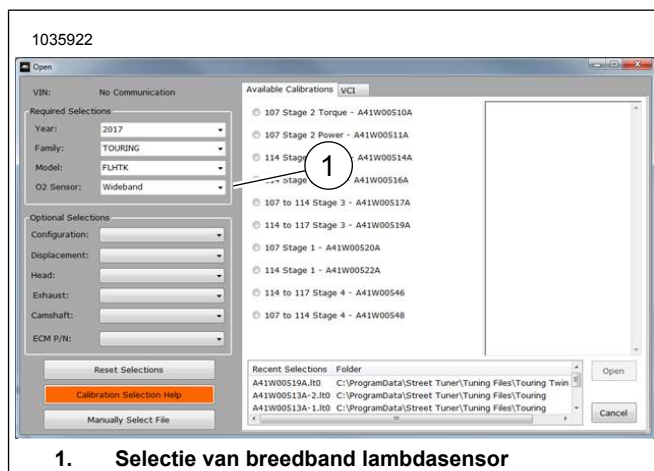
Afbeelding 37. Selectie van breedband lambdasensor
