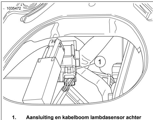
1. Aansluiting en kabelboom lambdasensor achter Afbeelding 38. Locatie achterste lambdasensor
