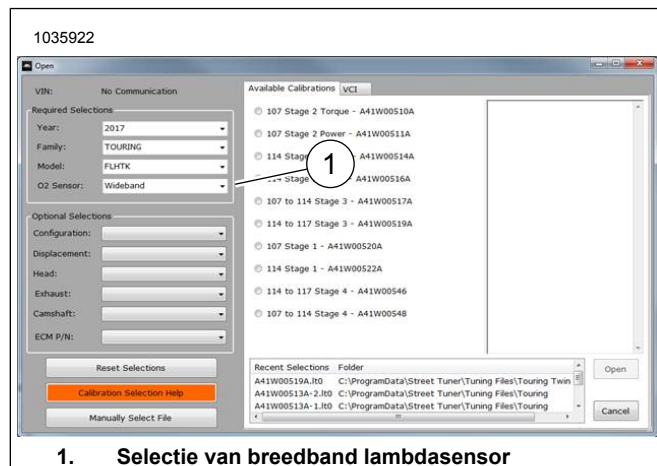
Afbeelding 17. Selectie van breedband lambdasensor
