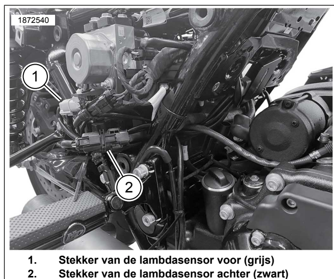
Afbeelding 4. Hoofdkabelboomaansluitingen van ATM
