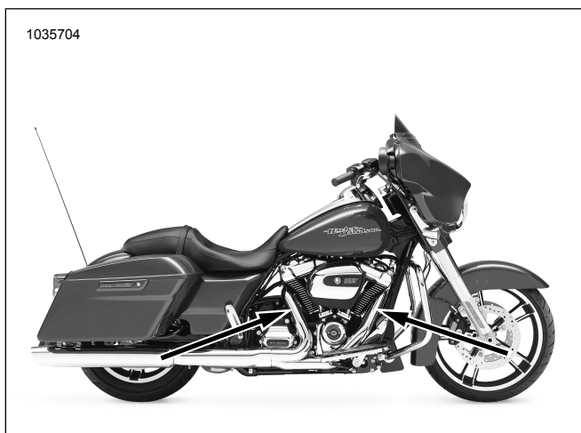
Afbeelding 11. Locaties van de lambdasensor (binnenzijde van uitlaatpijpen)
