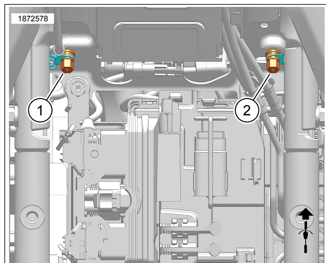
Afbeelding 6. Aardingsdraad geleiding
