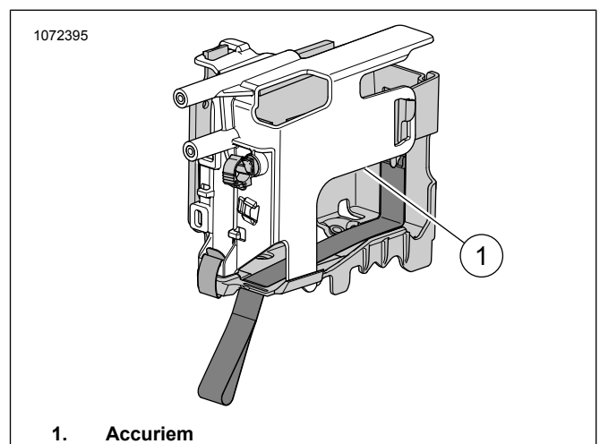
Afbeelding 19. Locatie accuriem
