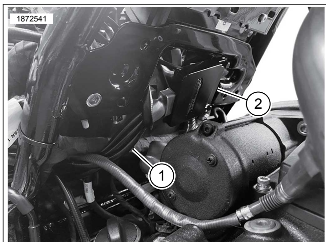
Afbeelding 5. Montagepositie van de ATM
