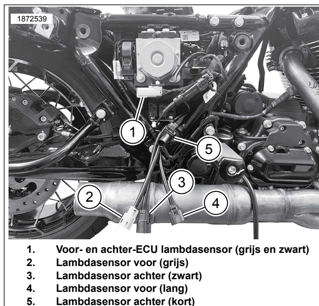
Afbeelding 3. Verloop van de grijze en zwarte stekkers van de kabelboom
