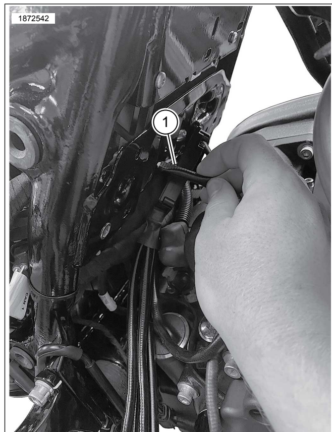
Afbeelding 6. Aardingsdraad geleiding
