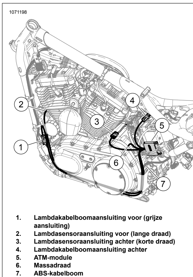
Afbeelding 50. Verloop ATM-kabelboom (plaatshouder)
