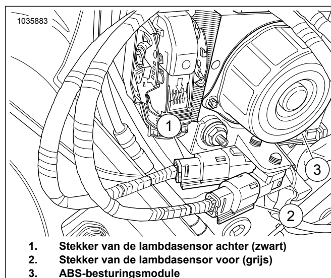
Afbeelding 13. Hoofdkabelboom aansluitingen van ATM
