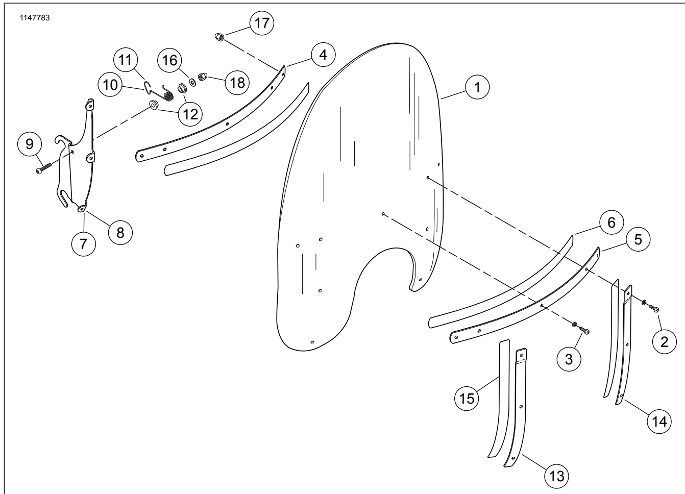
Afbeelding 1. Serviceonderdelen: Windscherm
