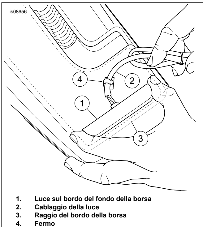
Figura 1. Installare la luce sul bordo del fondo della borsa
