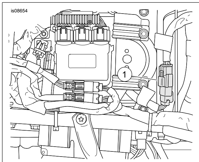
Figura 3. Connettore [7A] delle luci di marcia/arresto
