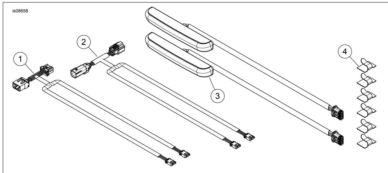
Figura 4. Parti di ricambio: Luci a LED di marcia/arresto/direzione ausiliarie per Electra Glo Stealth
