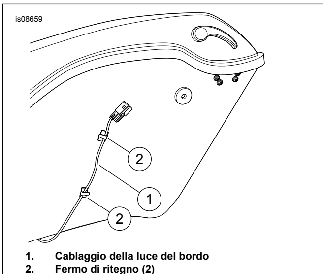
Figura 2. Conservare il cablaggio
