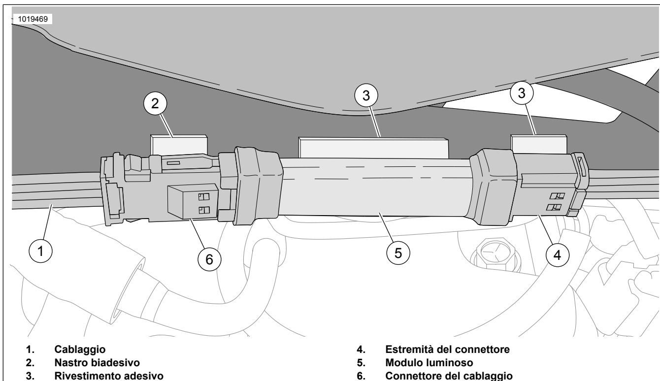
Figura 1. Modulo luminoso, connettori e nastro biadesivo
