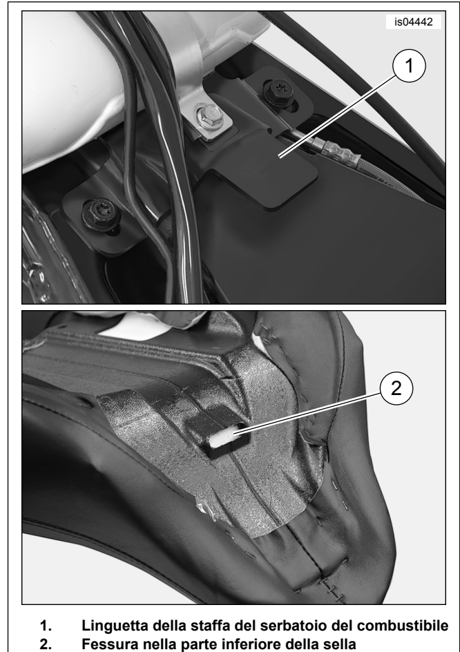
Figura 1. Montaggio anteriore della sella
