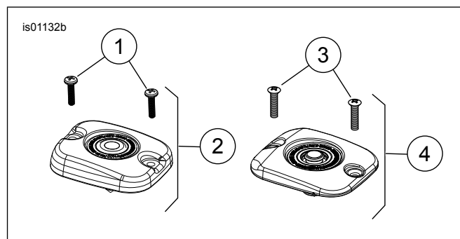
Figura 1. Parti di ricambio: Kit coperchio della pompa del freno
