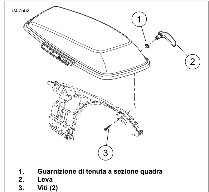
Figura 1. Gruppo leva
