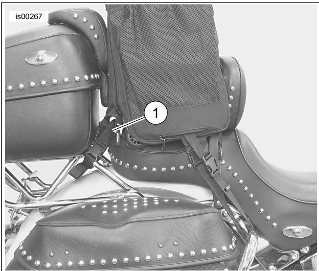
Figura 8. Configurazione cinghie No 3
