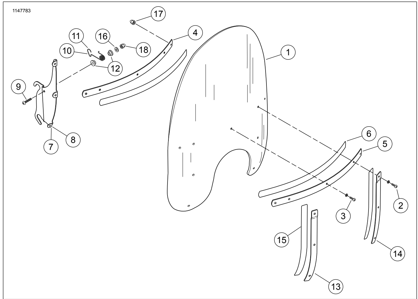
الشكل 1. قطع غيار الخدمة: مجموعة حاجب الريح
