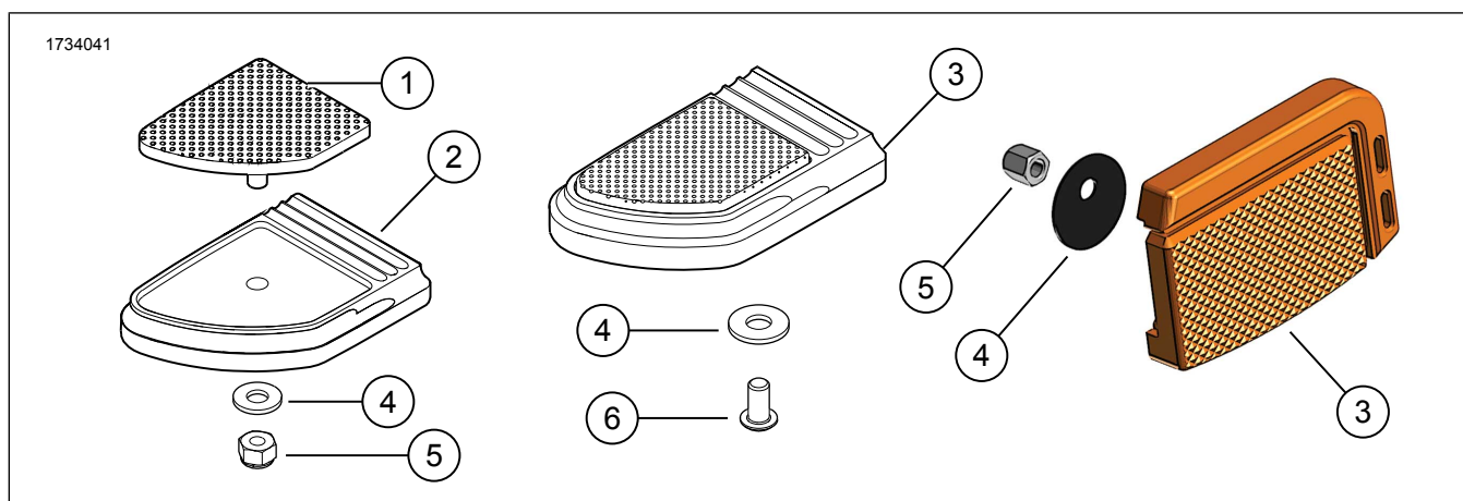
Rysunek 1. Zawartość zestawu: Zestaw nakładki na pedał hamulca
