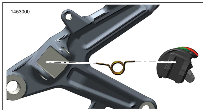
Rysunek 5. Orientacja sprężyny powrotnej - prawa
