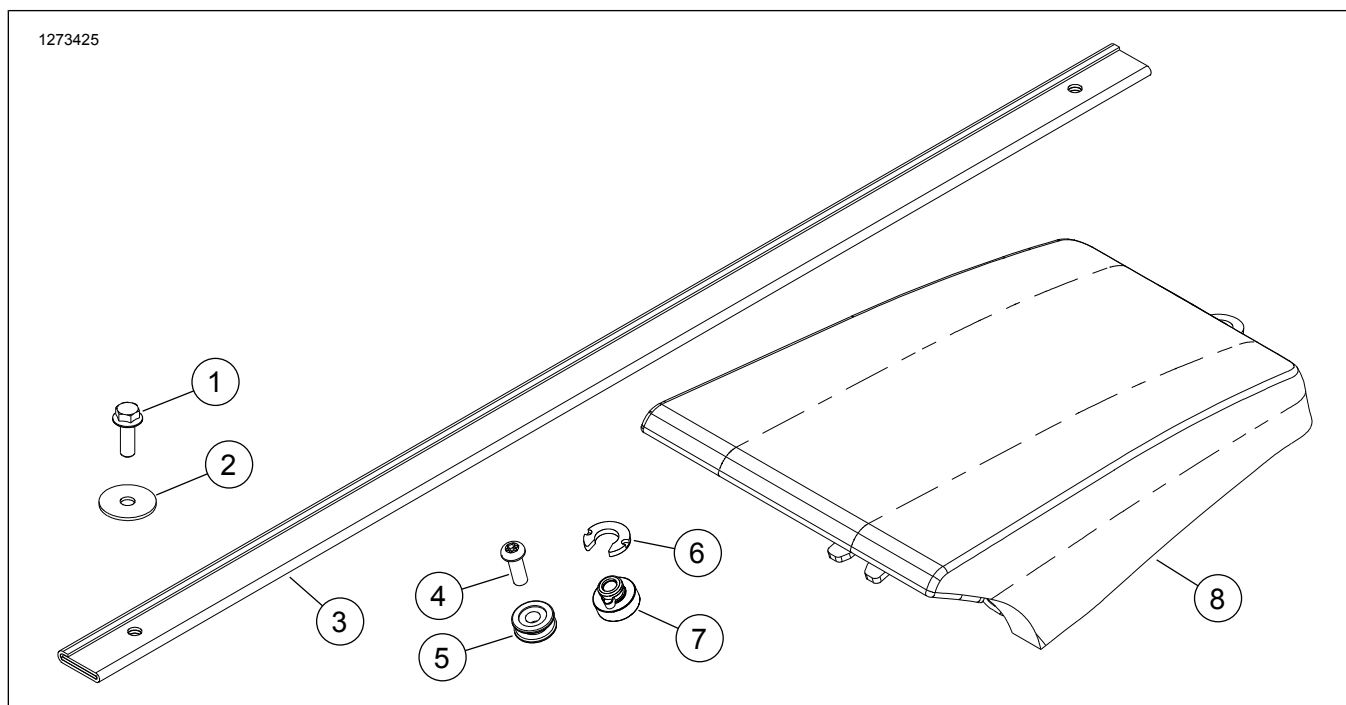
Figure 5. Pièces de rechange : Kit de selle de passager FXFB
