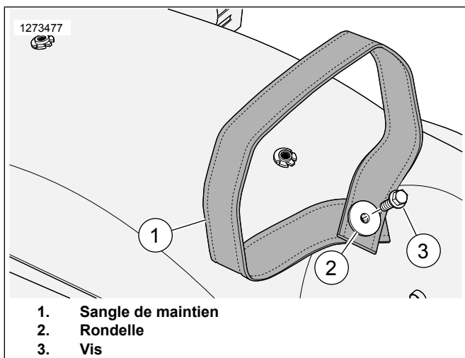
Figure 2. Sangle de maintien
