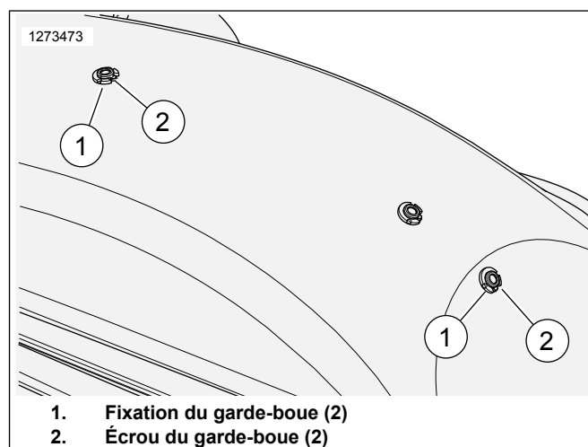
Figure 1. Fixation et écrou du garde-boue
