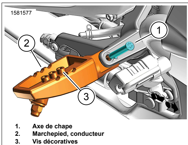
Figure 4. Installer l'ensemble de marchepied avec détente à ressort
