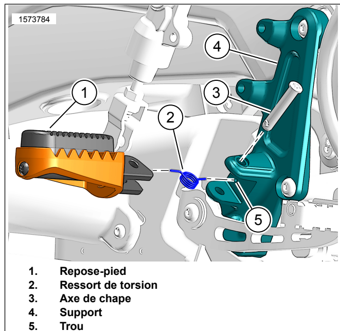
Figure 3. Retirer/installer l'ensemble de marchepied avec détente à ressort
