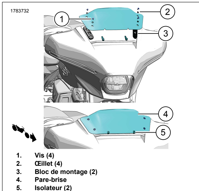
Figure 3. Installez le pare-brise coupe-vent
